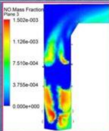
Розподіл концентрації оксидів азоту при трьохступеновому спалюванні вугілля
