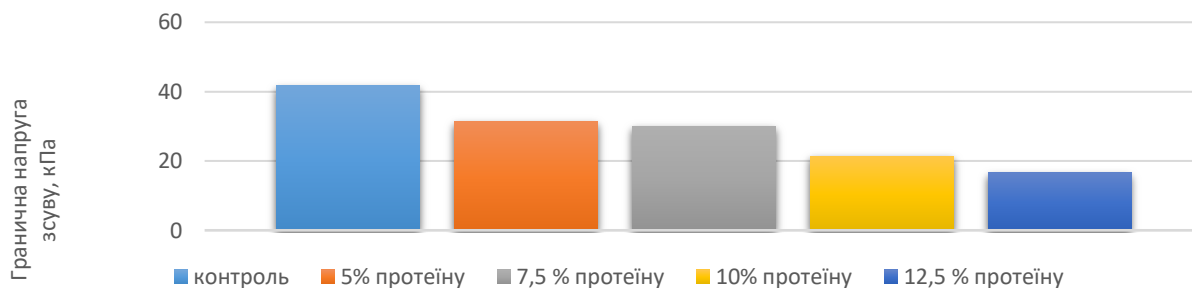
Рис. 3. Гранична напруга зсуву готових виробів
